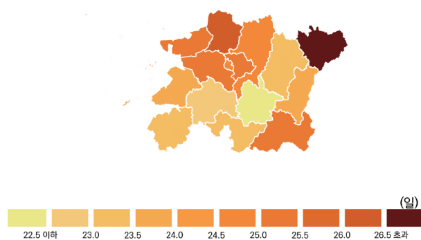
그림 3-4. 현재(2000-2019년) 전라북도 강수 관련 극한기후지수 분포(계속)
