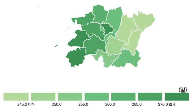
그림 3-2. 현재(2000-2019년) 전라북도 고온 관련 극한기후지수 분포(계속)
