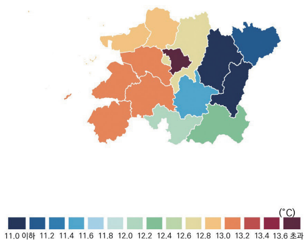
(c) 연평균 최저기온
