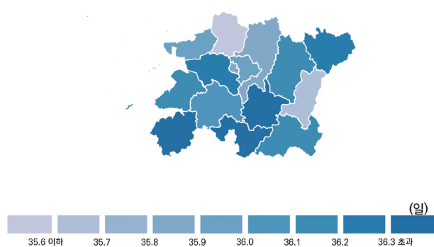
그림 3-3. 현재(2000-2019년) 전라북도 저온 관련 극한기후지수 분포
