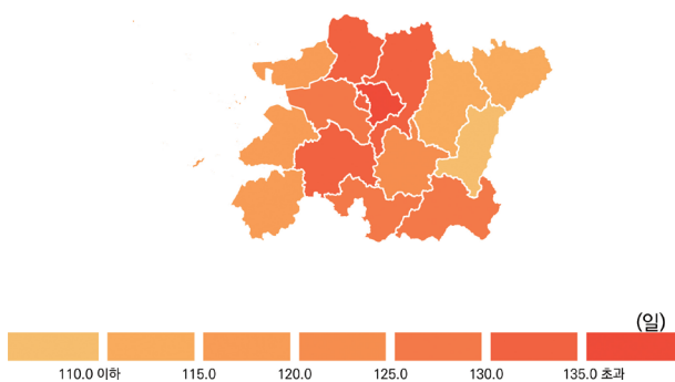
그림 3-2. 현재(2000-2019년) 전라북도 고온 관련 극한기후지수 분포
